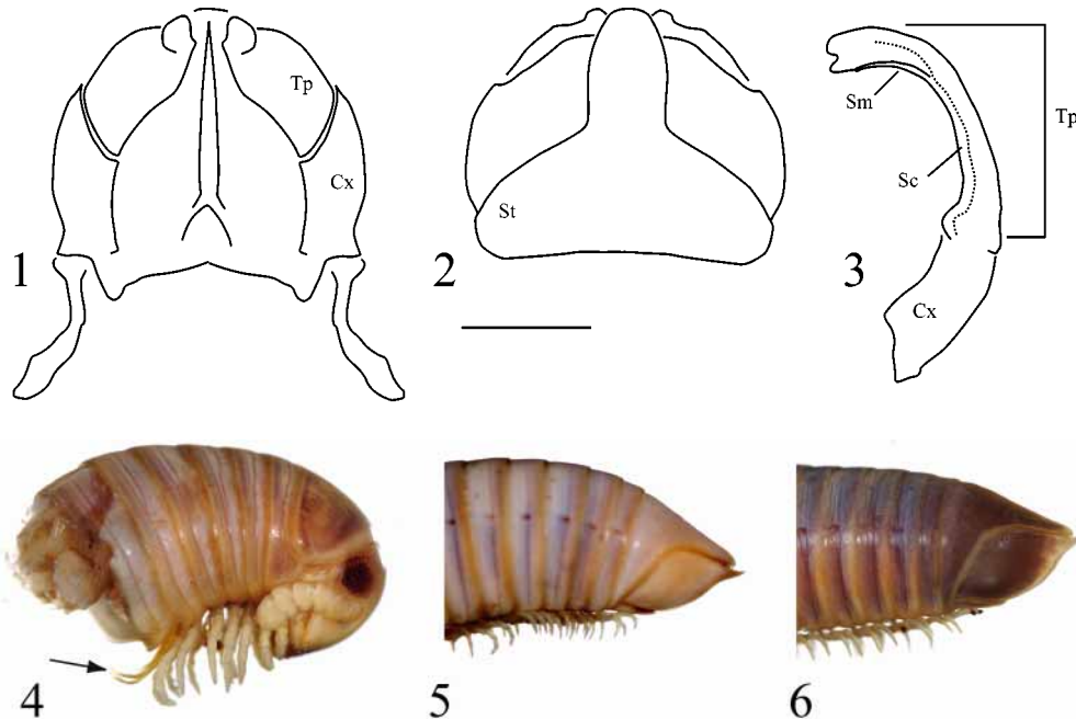
FIGURES 1-6. Oxygyge varicolor Silvestri, 1896. 1, anterior gonopod, posterior view. 2, anterior gonopod, anterior view. 3, left posterior gonopod. 4, lateral view of male anterior segments, arrow points to gonopods. 5, posterior segments, male. 6, posterior segments, female. [Scale bar = 1.0 mm (Figs. 1–3)]
