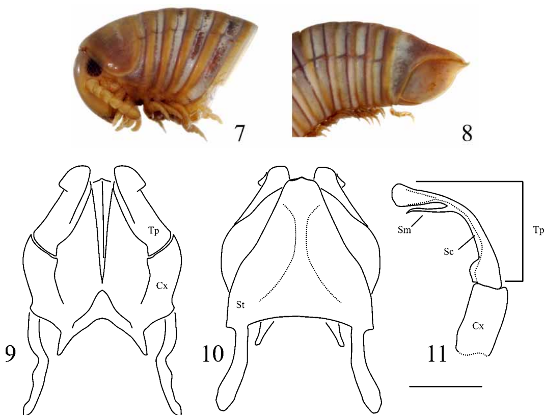
FIGURES 7–11. Oxygyge ferruginipes Chamberlin, 1922, male holotype. 7, lateral view of male anterior segments. 8, posterior segments, male. 9, anterior gonopod, posterior view. 10, anterior gonopod, anterior view. 11, left posterior gonopod. [Scale bar = 1.0 mm (Figs. 9–11)]
