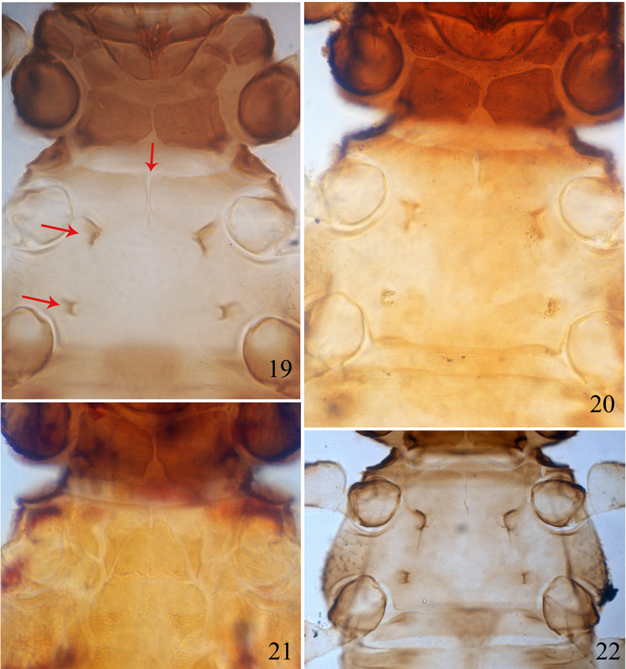
FIGURES 19–22. Mesoeusternum, meso- and metafurcae of Stephanothrips spp.: (19) S. austrinus sp. n.; (20) S. japonicus ; (21) S. kentingensis ; (22) S. occidentalis
