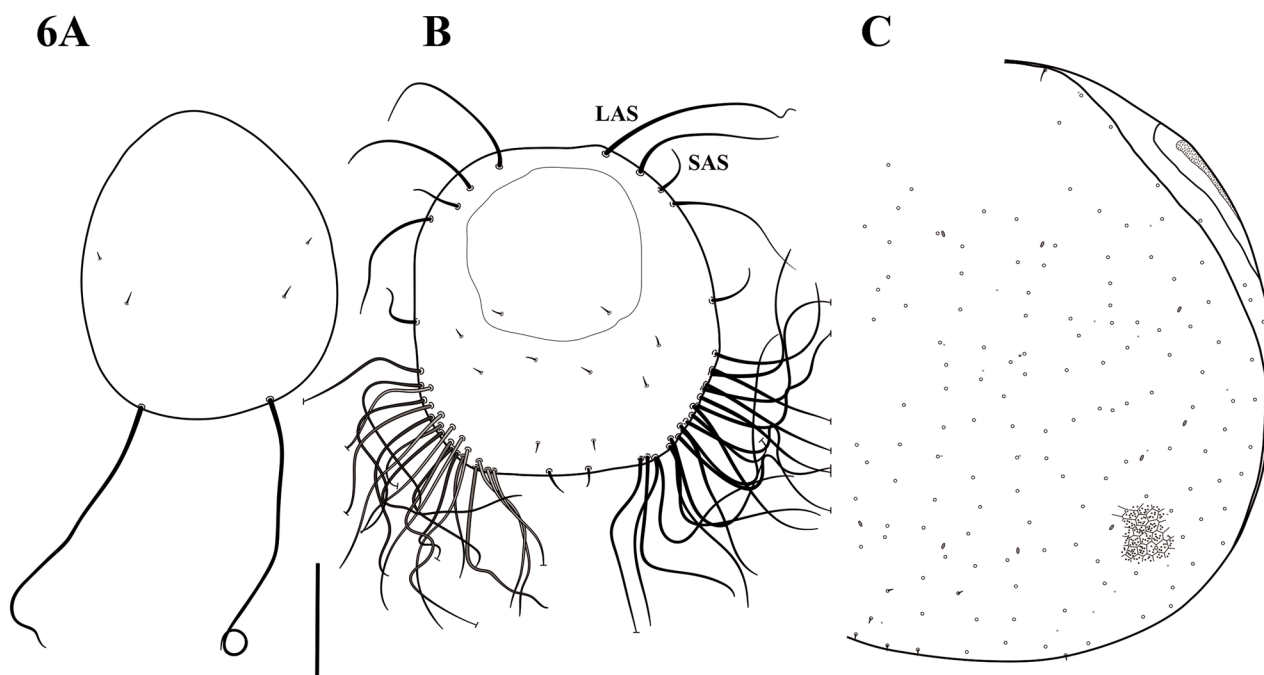
FIGURE 6. Philippinozercon makilingensis sp. nov., idiosoma, dorsal. A, Larva (OSAL 0118721); B, Protonymph (OSAL 0118723); C, Male (OSAL 0053267). Abbreviations: LAS, long anterior seta; SAS, short anterior seta. Scale bar A, B = 100 \mu m; C = 200 \mu m.
